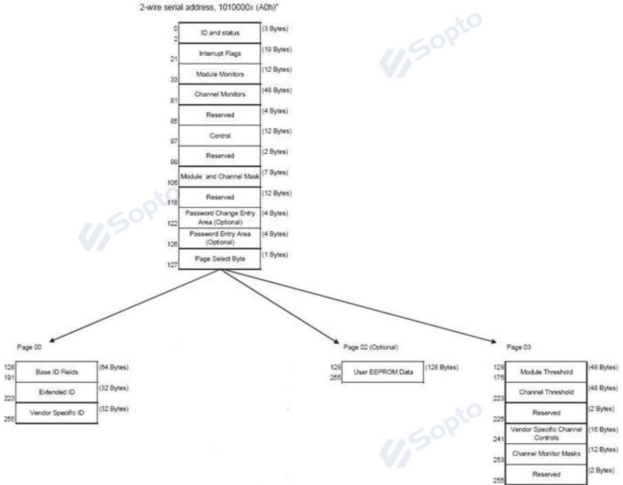
Figure4. QSPF Memory Map
